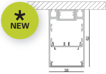
PLANO ES profiles page 540
